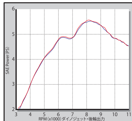
エアフィルター比較 左:ノーマル 右:SP武川製
