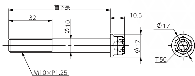
フランジ六角ボルト寸法図
