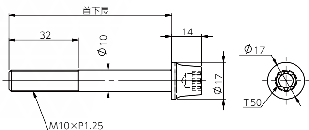
テーパークャップボルト寸法図
