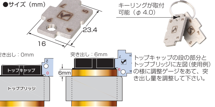
フロントフォーク組付け時の0位置合わせや突き出し量を変えたい時、0mmから7mmまでの1mm刻みで調整できるコンパクトな簡易ゲージです。
