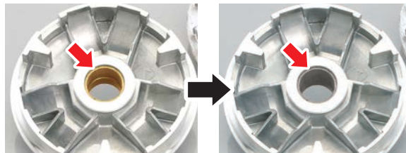
銅系焼結センターブッシュ (従来品)
