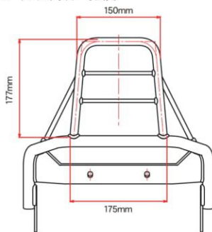
ツーリングキャリア 寸法図
