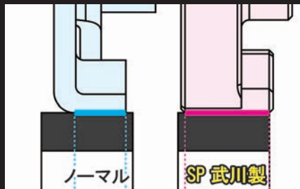
プッシュロッドヘッドへの接地面積を増やし、ゴムの破損を軽減します。
