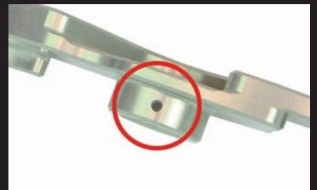
オイルの潤滑を行うオイル穴を装備
