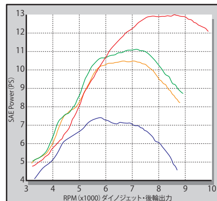
FIコンTYPE-e(インジェクションコントローラー)
