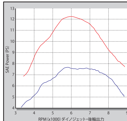
テスト車両:CT125(JA55) ■Sステージαボアアップキット181cc+スポーツマフラー ■ノーマルエンジン+ノーマルマフラー
